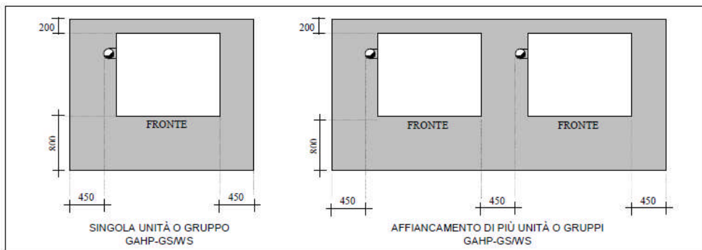
Figura 2 - Distanze di rispetto per unità GS/WS fino a un massimo di 5 unità
