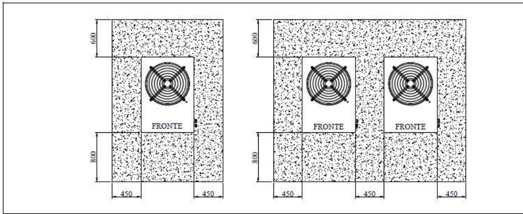
Figura 1 - Distanze di rispetto per unità GAHP e GA fino a un massimo di 5 unità
