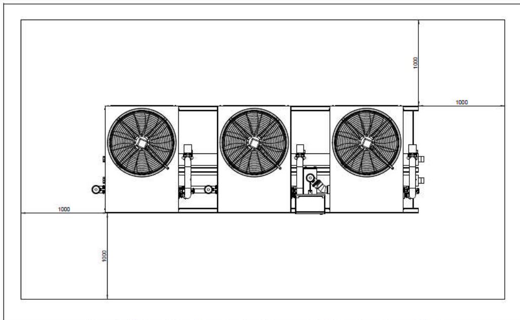
Figura 3 - Distanze di rispetto per singole unità preassemblate in configurazione multi-link
