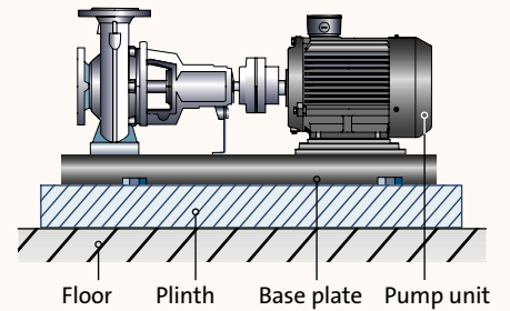
Fig. 2.1.7: Plinth
