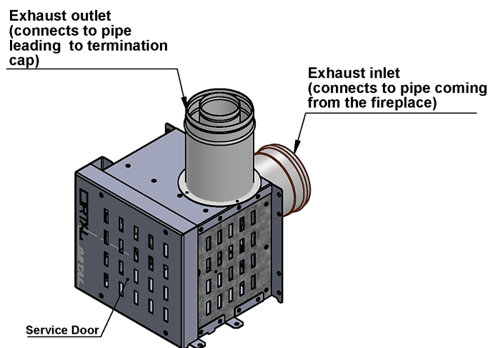
Inline Power Vent Fan Exhaust Inlet & Outlet
